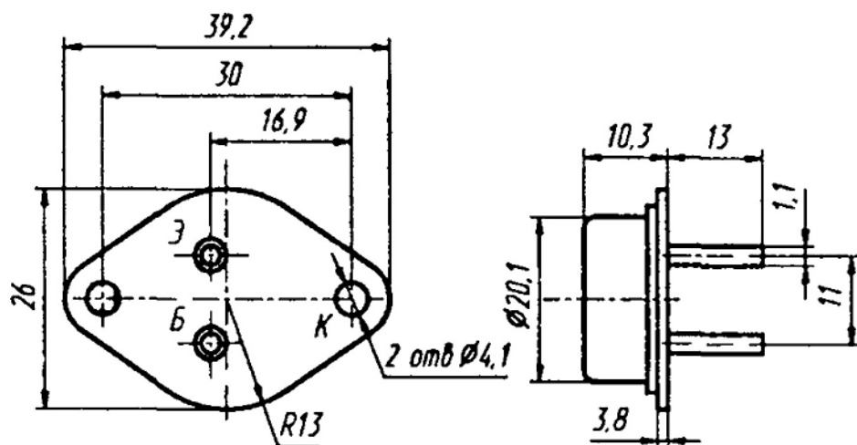
2Т818(А-В), КТ818(АМ-ГМ)
