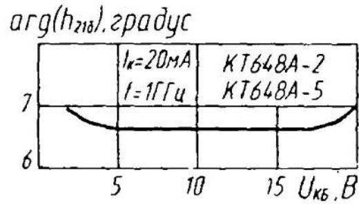
Зависимость аргумента коэффициента передачи тока на высокой частоте от напряжения коллектор—база
