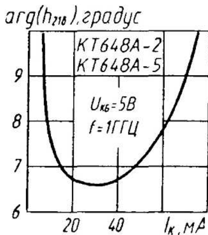
Зависимость аргумента коэффициента передачи тока на высокой частоте от тока коллектора
