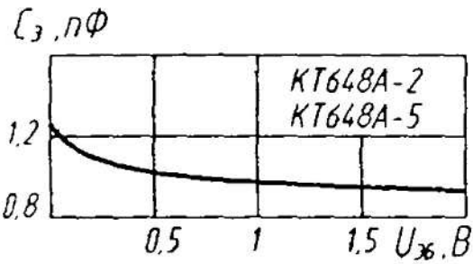
Зависимость емкости эмиттерного перехода от напряжения эмиттер—база
