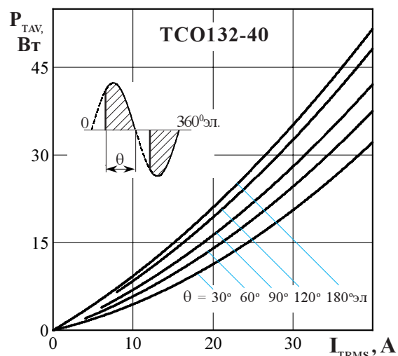
Рисунок 4 - Зависимость средней мощности потерь P_{TAV} от действующего значения тока I_{TRMS} в открытом состоянии синусоидальной формы частоты f = 50 Гц
